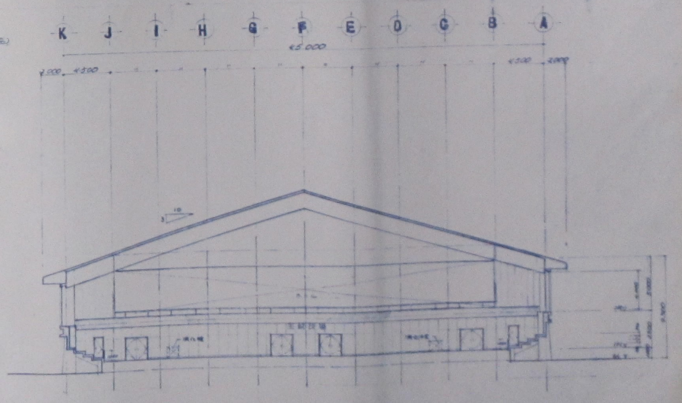
A-K 断面图 SCALE 1:100
