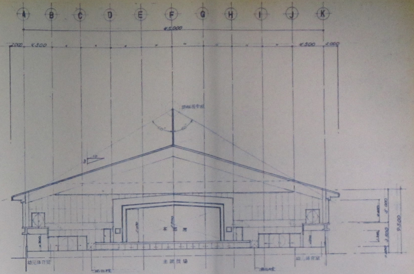
A-K 断面图 SCALE 1:100
