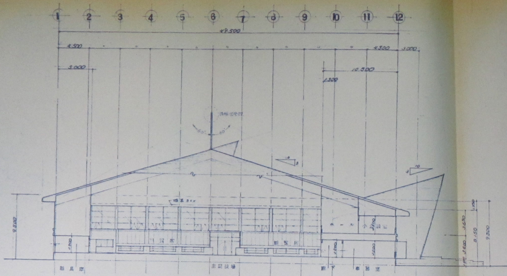
1-12 断面图 SCALE 1:100
