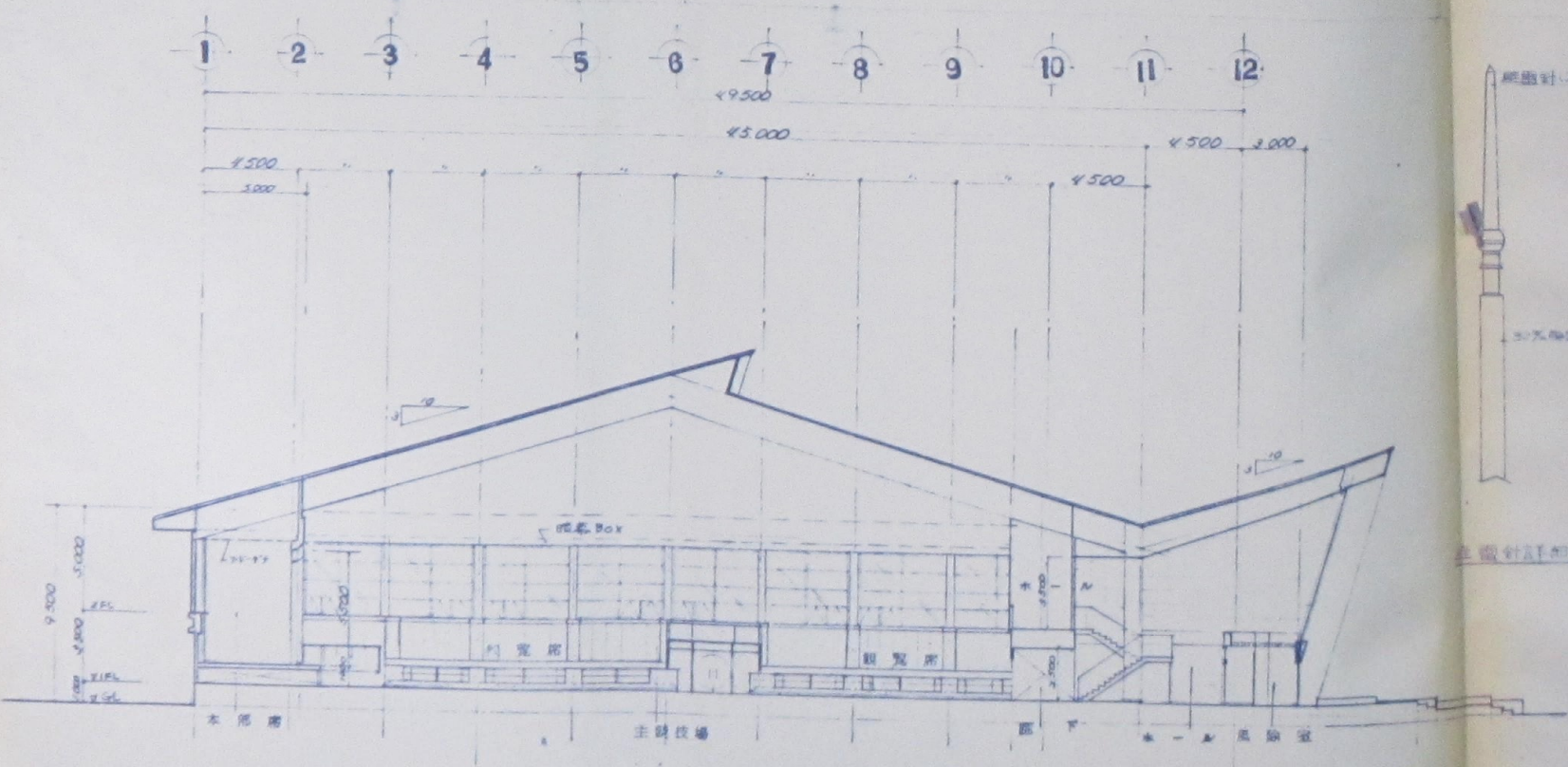
1-12 断面图 SCALE 1:100
