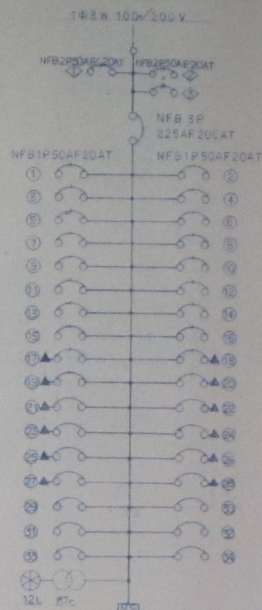
L-2 分電盤
