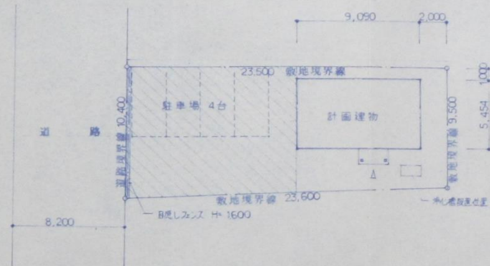
配置図 S=1/200
