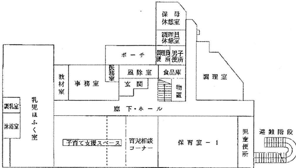
1 階平面図
