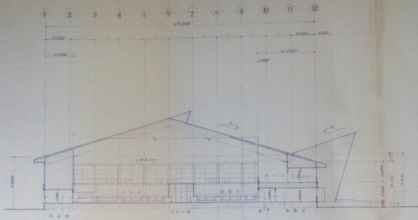
1-12 斷面圖 SCALE 1:125
