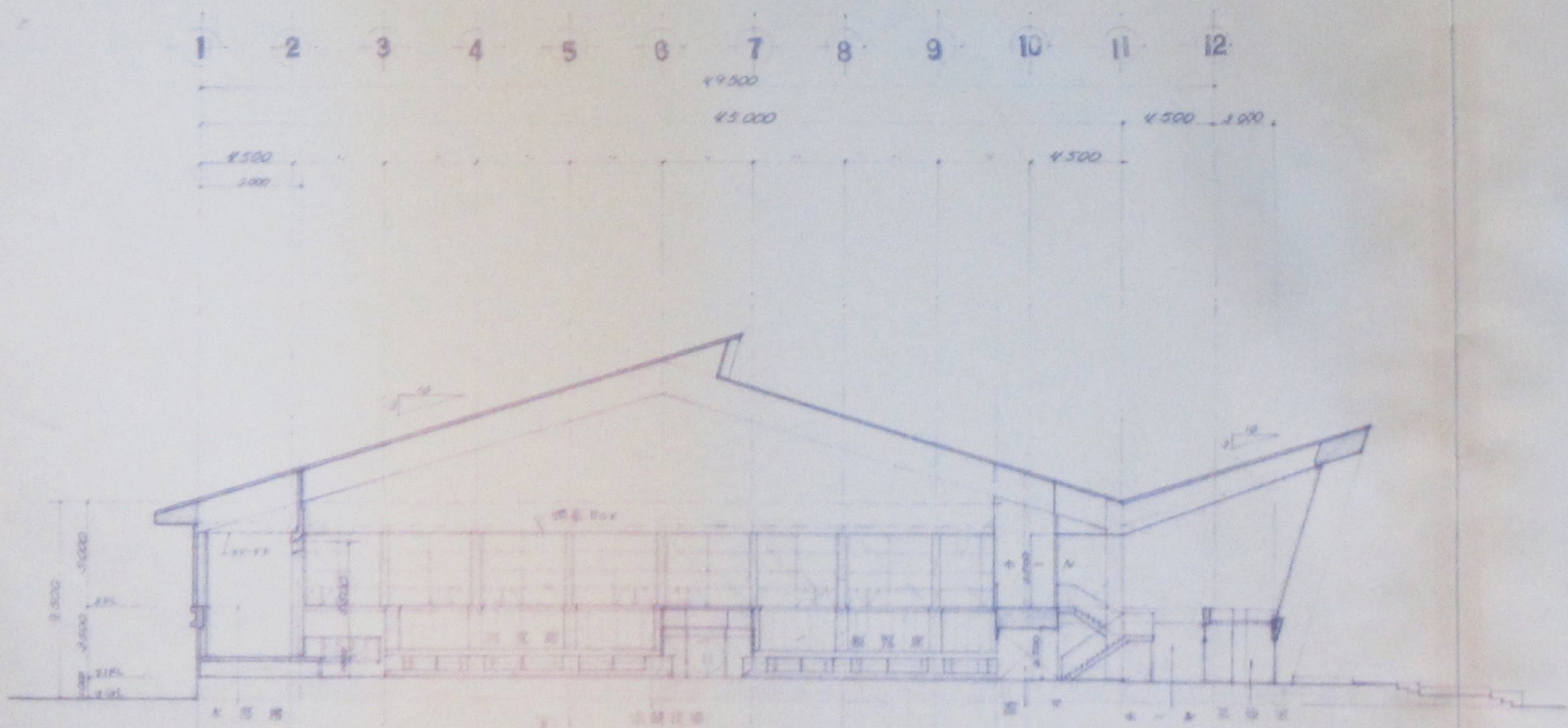
1-12 斷面圖 SCALE 1:125
