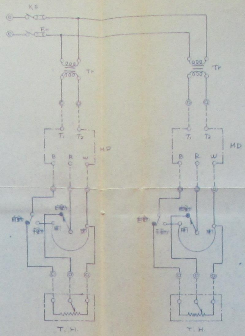
電動機制御盤内配線図
